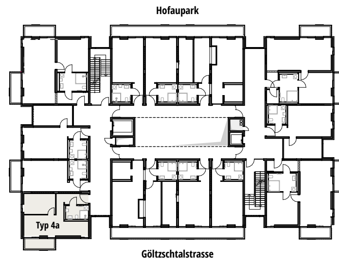
ÜBERSICHTSGRUNDRISS 1.-4. OBERGESCHOSS M 1:500
