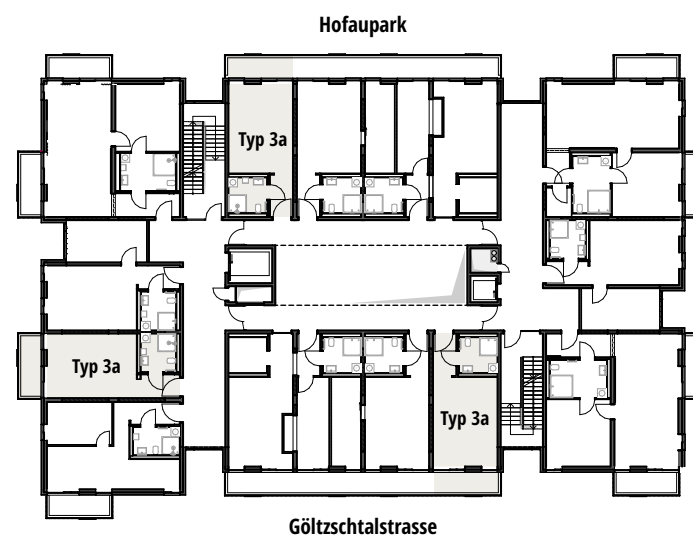
ÜBERSICHTSGRUNDRISS 1.-4. OBERGESCHOSS M 1:500
