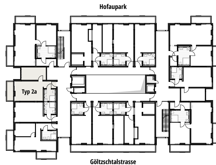
ÜBERSICHTSGRUNDRISS 2.-4. OBERGESCHOSS M 1:500
