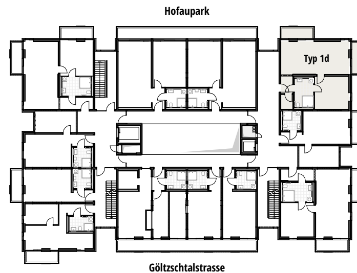
ÜBERSICHTSGRUNDRISS 3.-4. OBERGESCHOSS M 1:500
